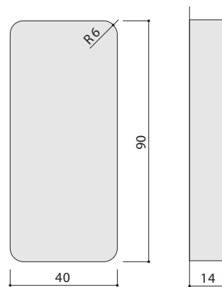
PC-210切欠き寸法（角R付）
