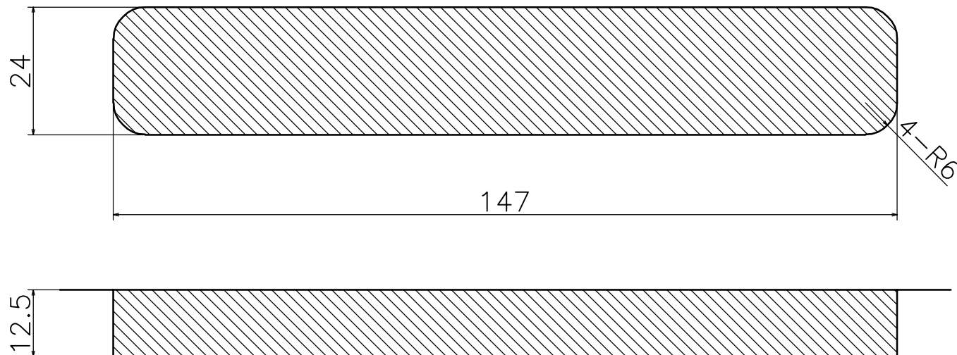
PC-303切欠き寸法（角R付）
