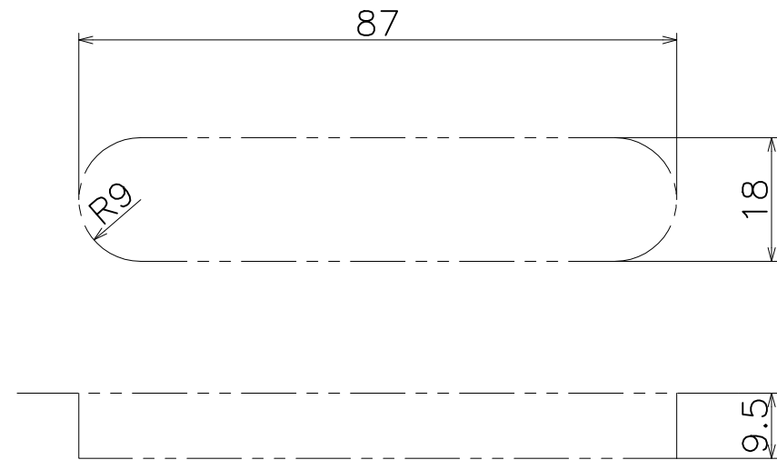
切欠図 (S=1:1)
