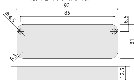
PC-143切欠き寸法（角R付）
